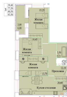
1 ЭТАЖ
